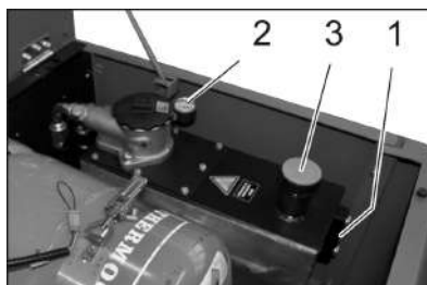
1 Vizor 2 Manometru 3 Capac de închidere, orificiu de umplere a uleiului
