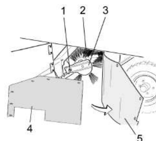
1 Vis de fixation du logement de la brosse de balayage
