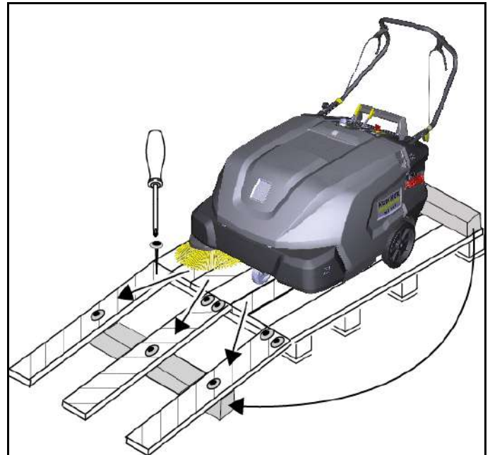
Kuva: Purkuluisikan rakentaminen
