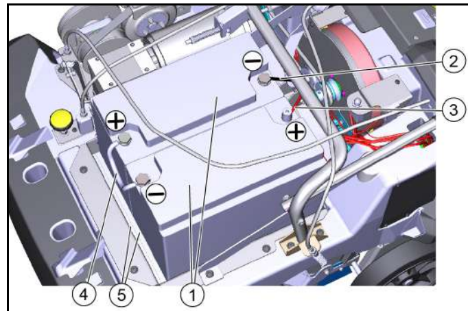
Kuva: Akkujen asentaminen ja liittäminen
