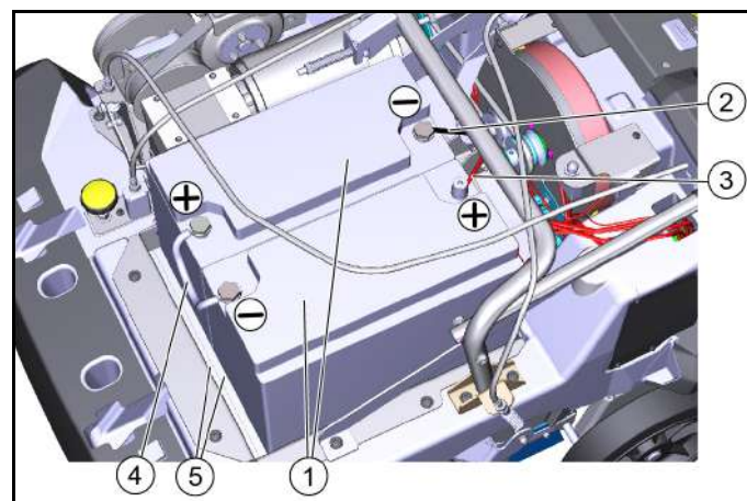
Figura: Montaje y conexión de las baterías
