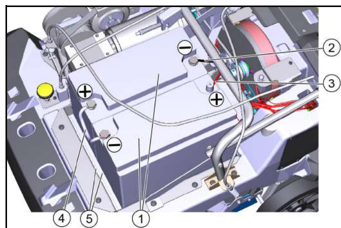
Figur: Montering og tilslutning af batterierne
