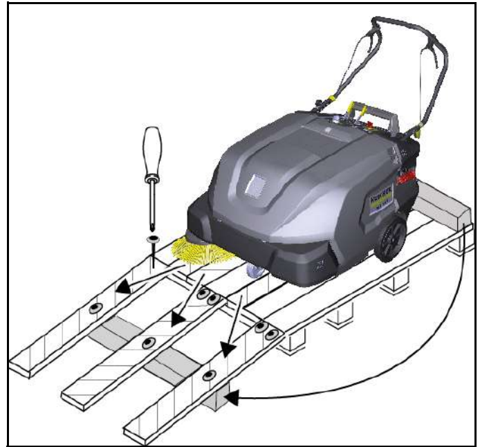
Figura: Creazione di una rampa di discesa
