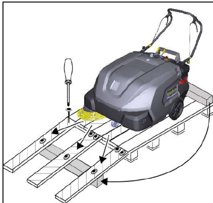
Pav.: Nuvažiavimo platformos montavimas
