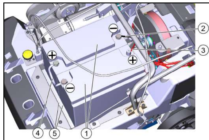
Figure : Montage et connexion des batteries
