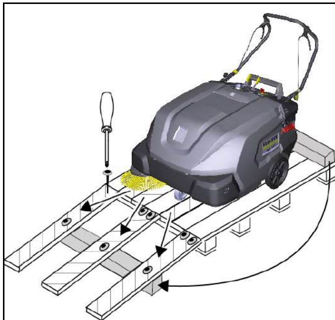
Slika: Izgradnja dovozne rampe
