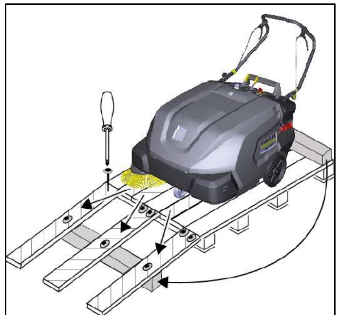
Figura: Construcción de una rampa hacia abajo
