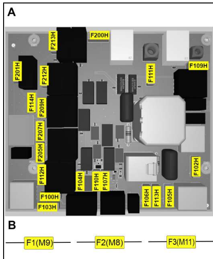
A: Fusibles del control electrónico
